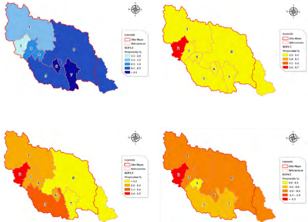
Figura 9. Proyecciones de cambio para precipitación (arriba) y temperatura (abajo) para dos escenarios de cambio climático RCP 4.5 (izquierda) y RCP 8.5 (derecha) para el periodo de 2011-2040 para la cuenca Alto Mayo. Los resultados se presentan en porcentaje, es decir, la variación media de la variable precipitación en relación con el periodo de base (1981-2010).).
