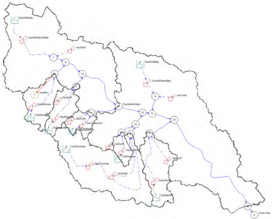
Figura 12. Porcentaje de cambio de los caudales mensuales por subcuencas respecto al escenario base (histórico).
